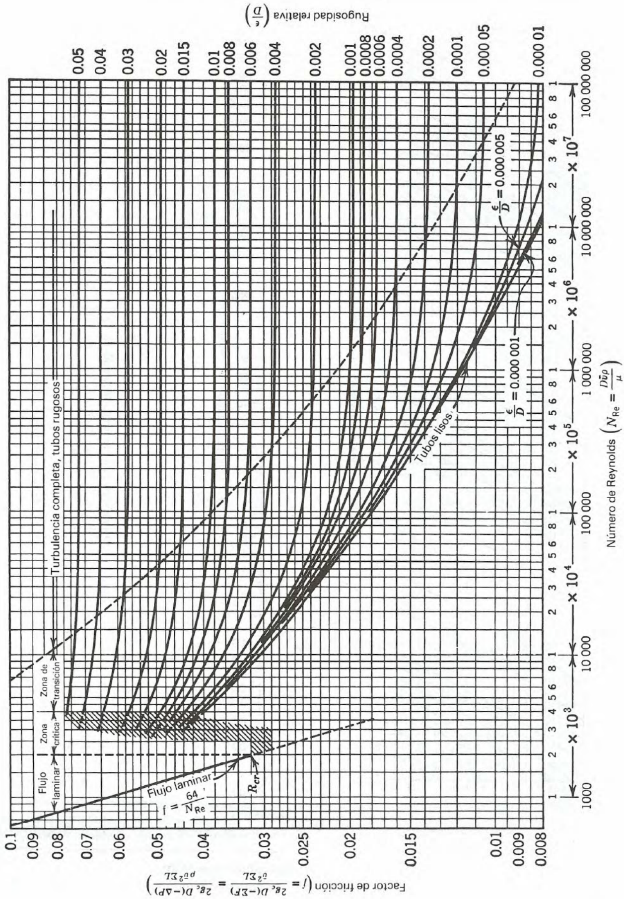
Apéndice C-3 Factor de fricción en función del número de Reynolds con la rugosidad relativa como parámetro [Moody, L. F., Trans. ASME , 66, Págs. 671-84(1944); Por cortesía de ASME.]
