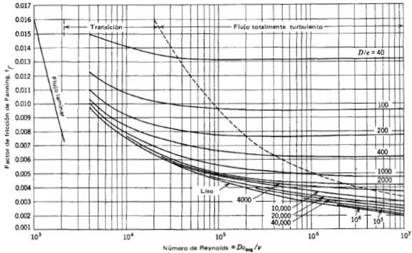
Figura 14.1 El factor de fricción de Fanning en función de Re y D/e .
