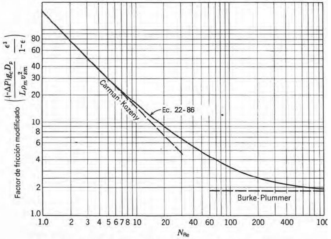
Fig. 22-30 Caída de presión para el flujo a través de lechos empacados.
