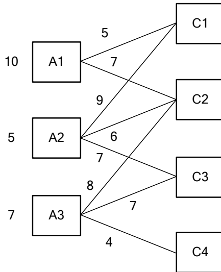
Figura 1: Sistema de distribución de una compañía.
