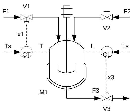
Figura 1: Tanque mezclador.
