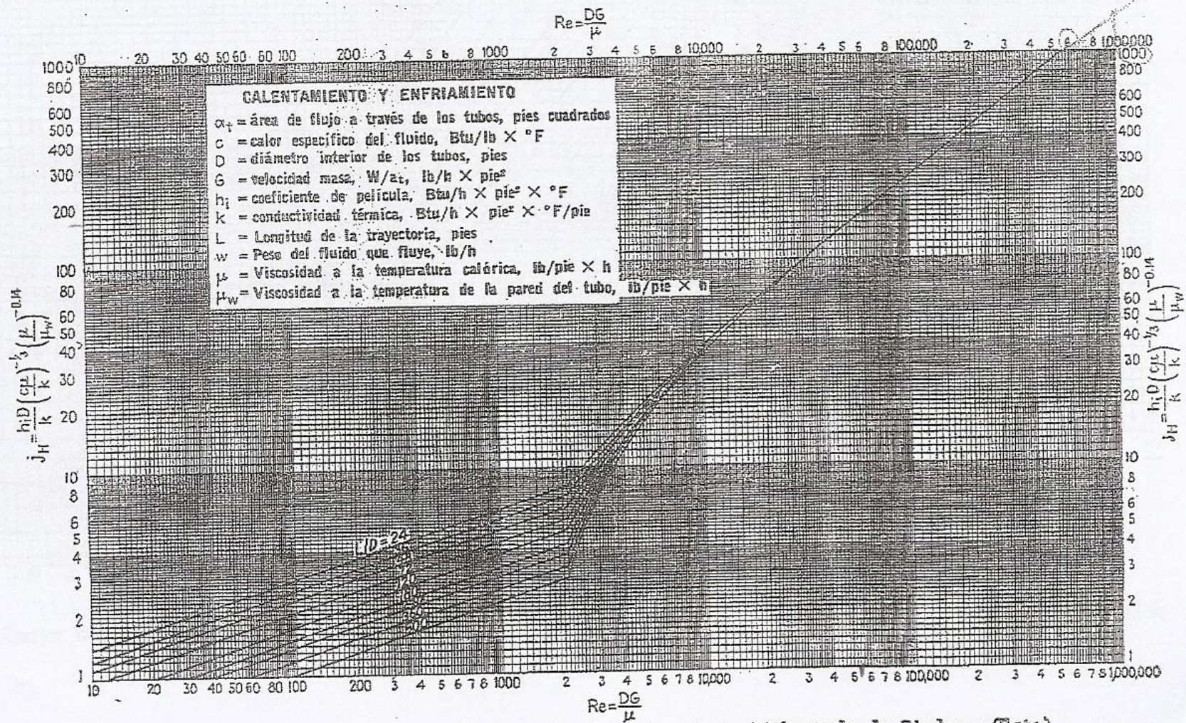
Curva de transferencia de calor lado de tubos. (Adaptada de Sieder y Tate)
