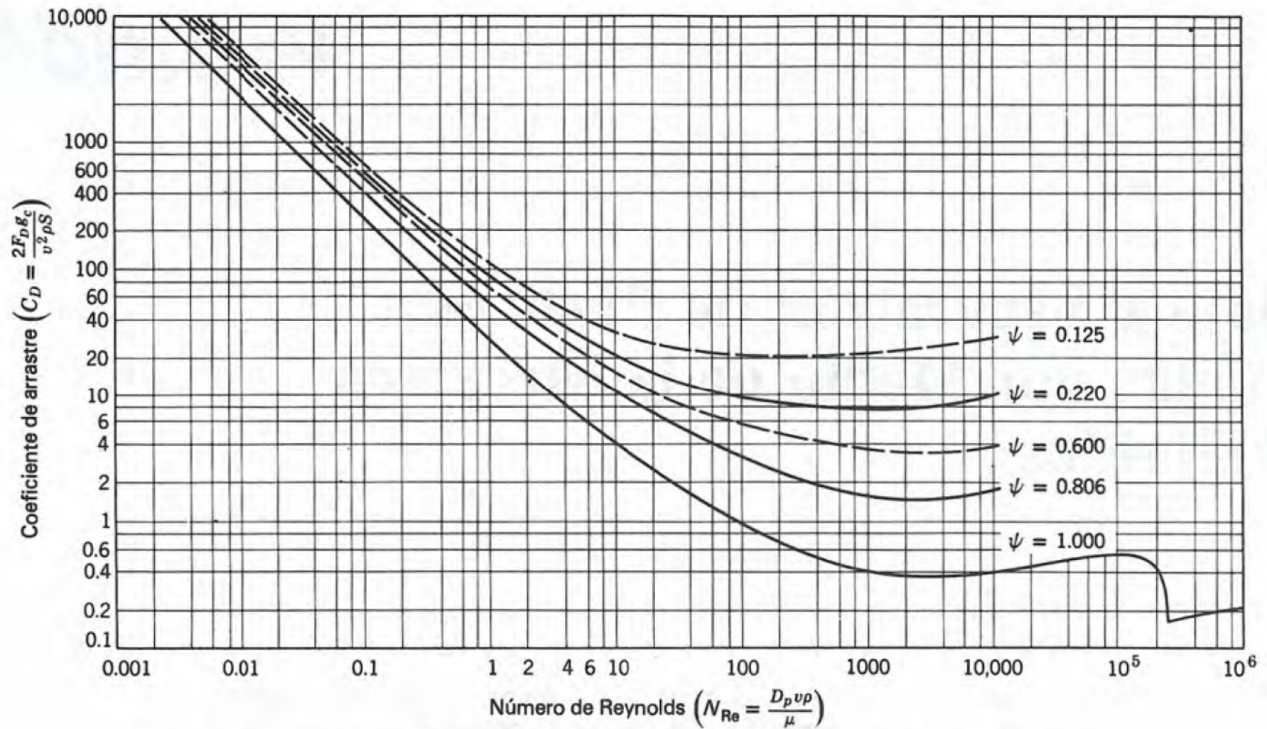
Fig. 22-1a Coeficiente de arrastre en función del número de Reynolds (60). (Con per-
