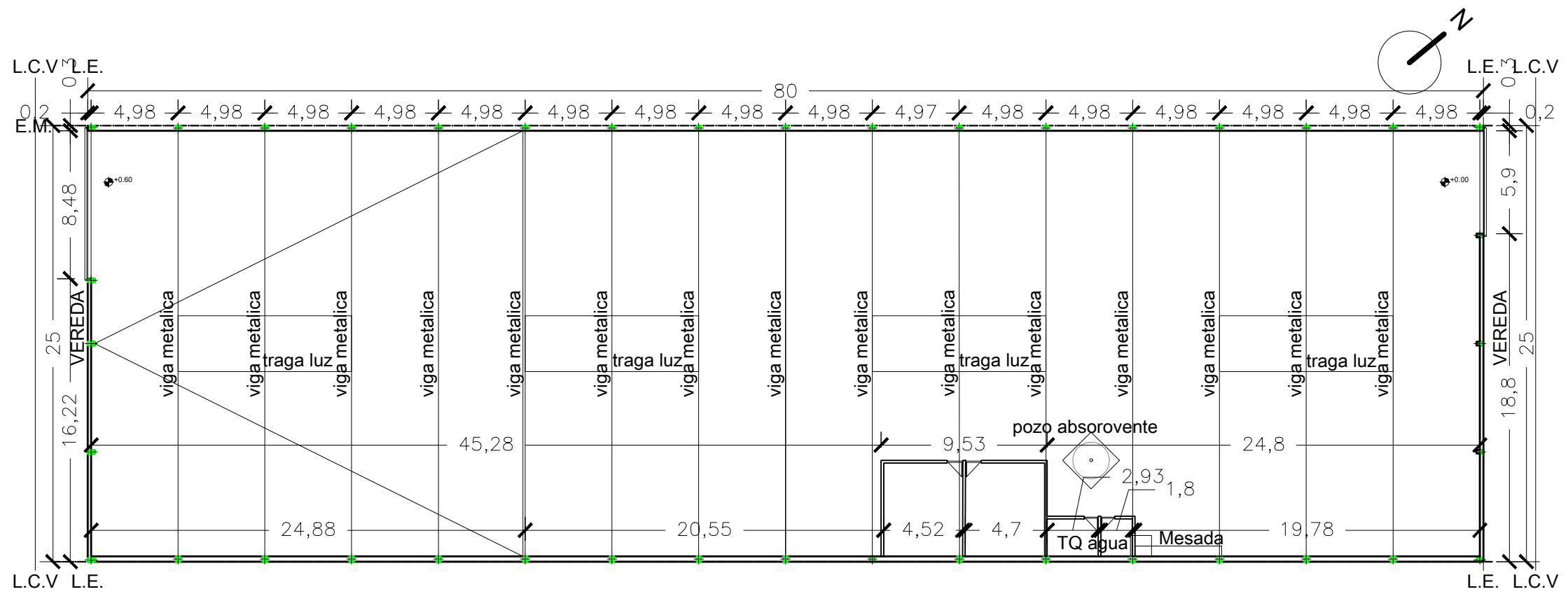
ESQUEMA PLANO PLANTA RELEVAMIENTO 1:500
