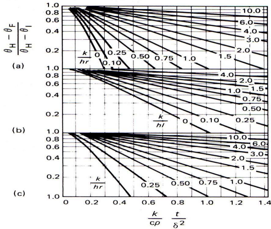
Diagrama para la transmisión de calor (a) esfera; (b) paralelepípedo; (c) cilindro. (Según Henderson y Perry (1955))
