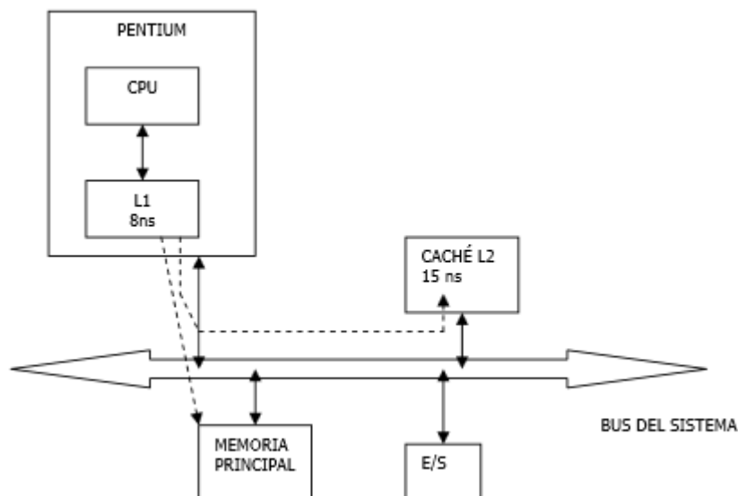
Figura 12. Conexionado paralelo.
