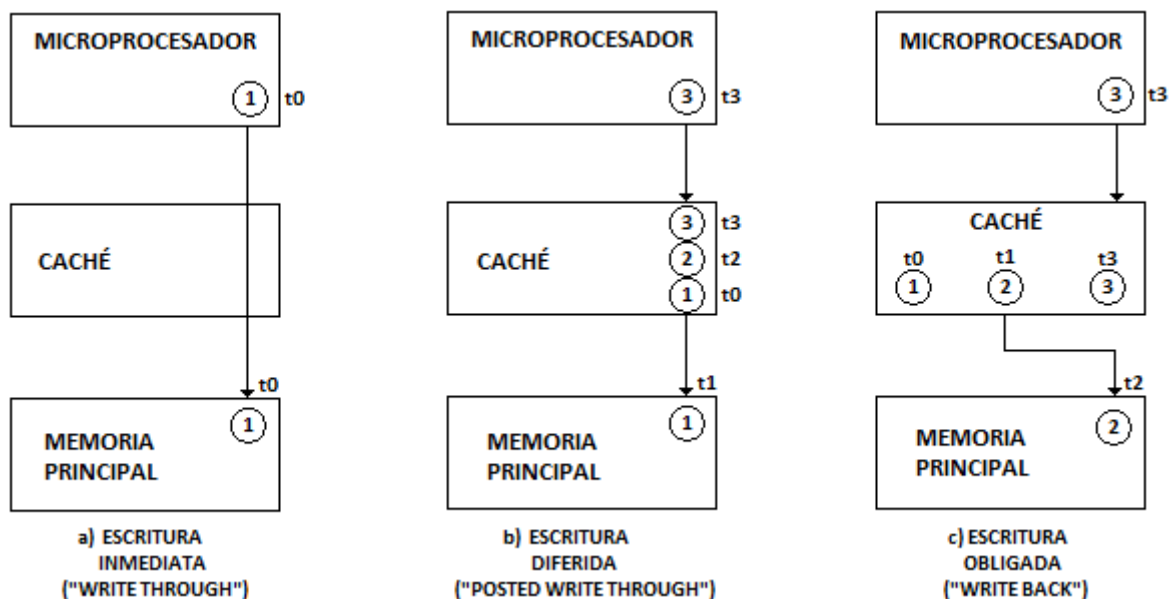
Figura 9. Tres métodos de actualización de la memoria principal de un subsistema caché.
