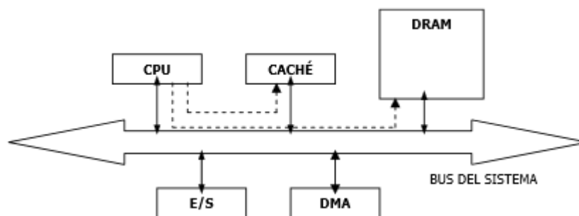
Figura 4. Conexión en paralelo.
