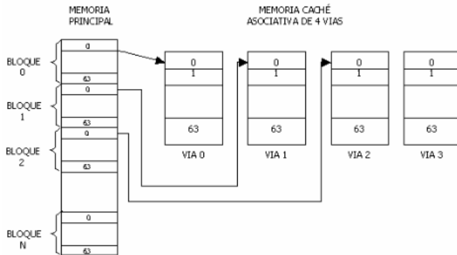
Figura 8. Organización asociativa de "N" vías de la memoria caché.
