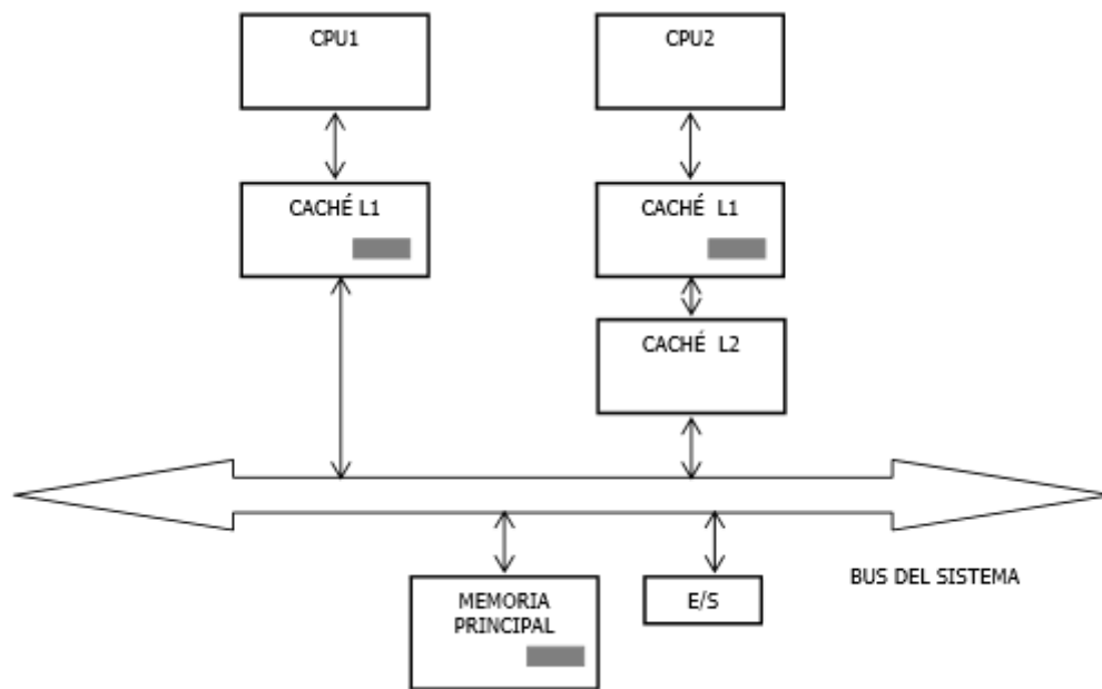
Figura 10. Multiprocesador con más de una caché.
