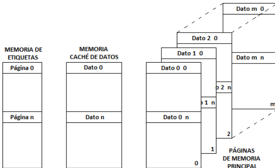
Figura 7. Organización asociativa de una sola vía de la memoria caché.
