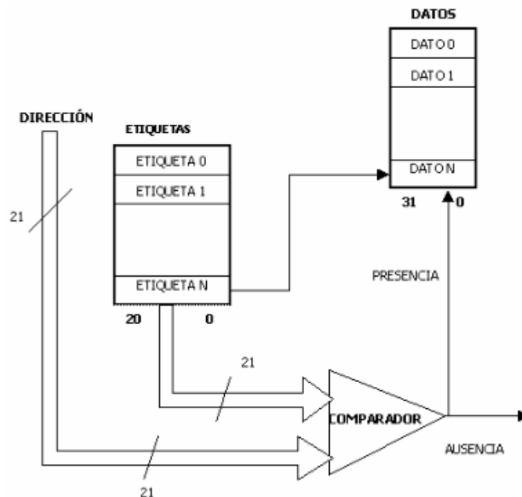
Figura 2. Principio de funcionamiento de la caché.
