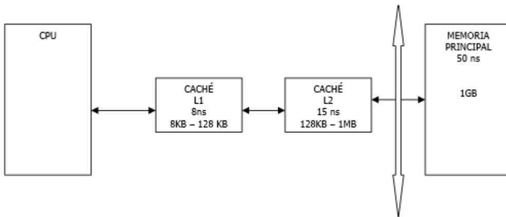
Figura 11. Utilización de cachés de primer y segundo nivel.
