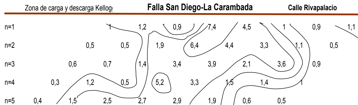
Fig 2.27. Sección de isorresistividades en una falla de tensión
