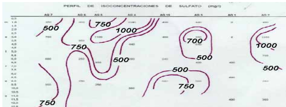
Fig 2.20. Perfiles de Potencial Natural y configuración de sulfatos
