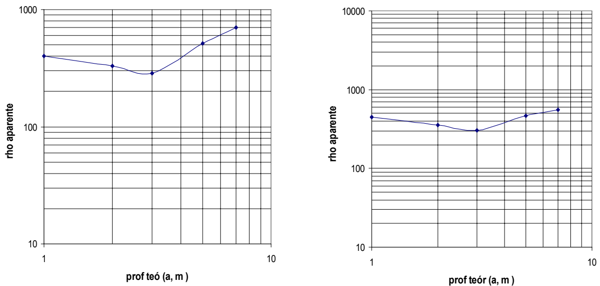
Fig 2.23. Curvas de resistividad aparente, AB/2-Ω-m
