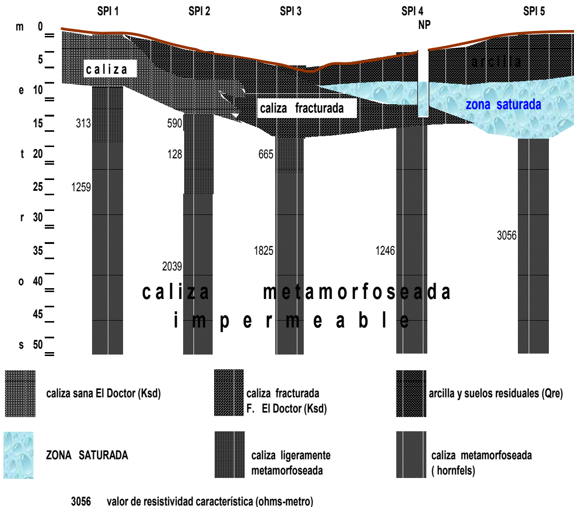
Fig 2.26. Sección geoelectrica interpretada
