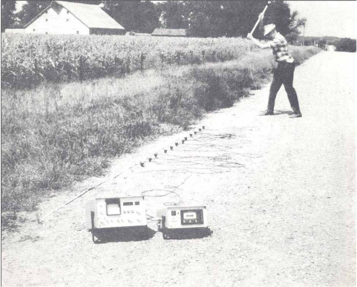
Fig 3.4. Tendido sísmico característico
