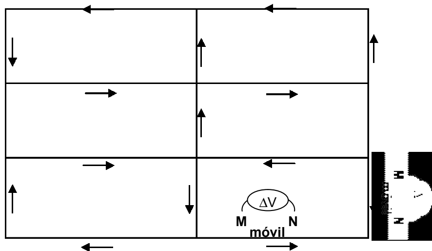
Fig 2.15. Método de Gradientes para medir el SP
