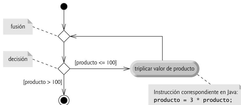
Fig. 4.6 | Diagrama de actividad de UML de la instrucción de repetición while .
