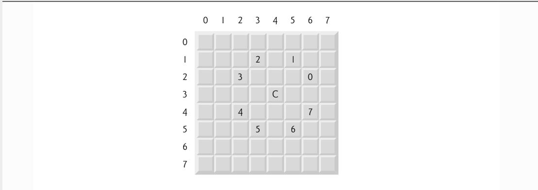
Fig. 7.30 | Los ocho posibles movimientos del caballo.
