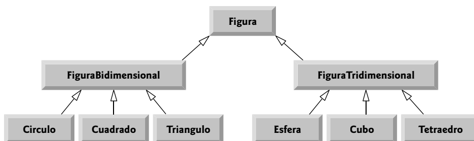
Fig. 9.3 | Diagrama de clases de UML de la jerarquía de herencia para Figuras.
