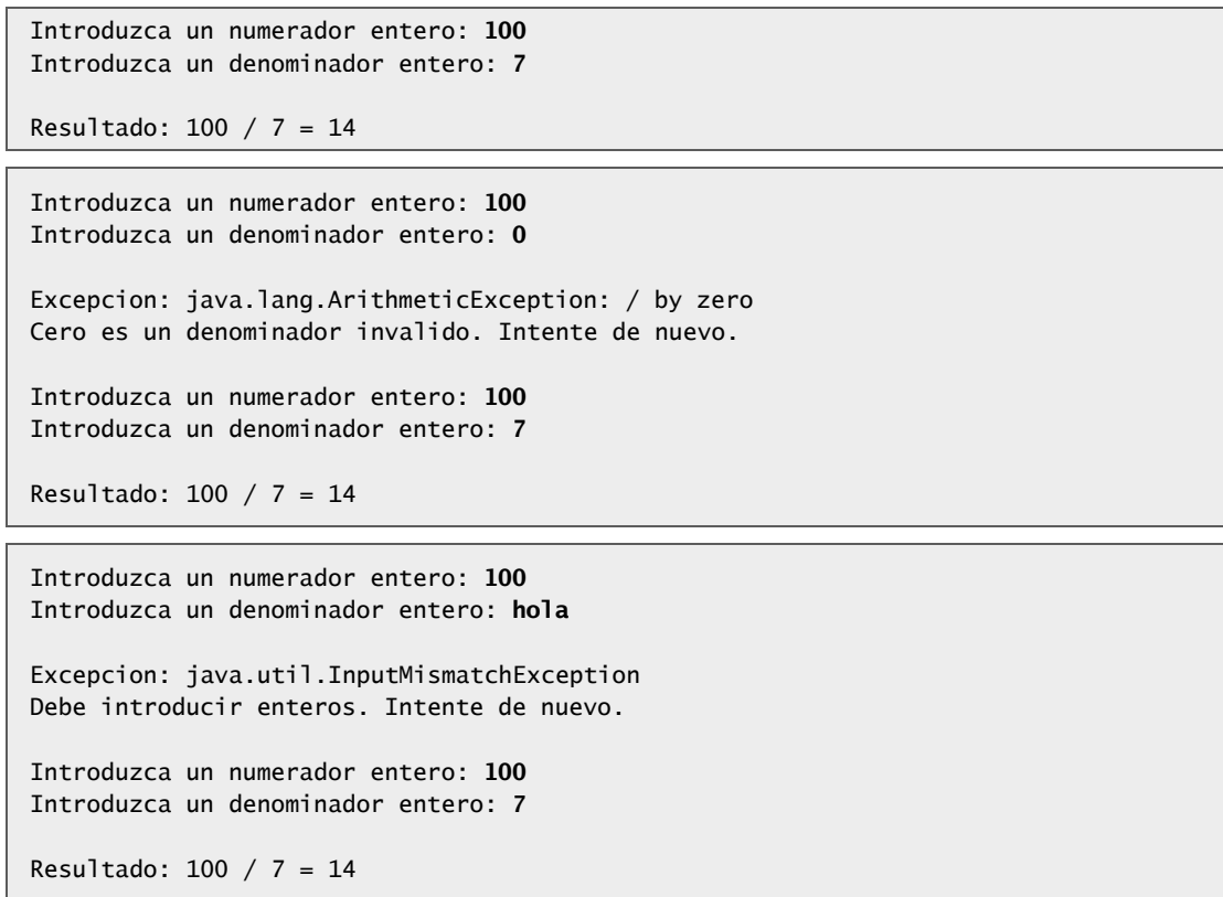
Fig. 11.3 | Manejo de excepciones ArithmeticException e InputMismatchException (parte 2 de 2).
