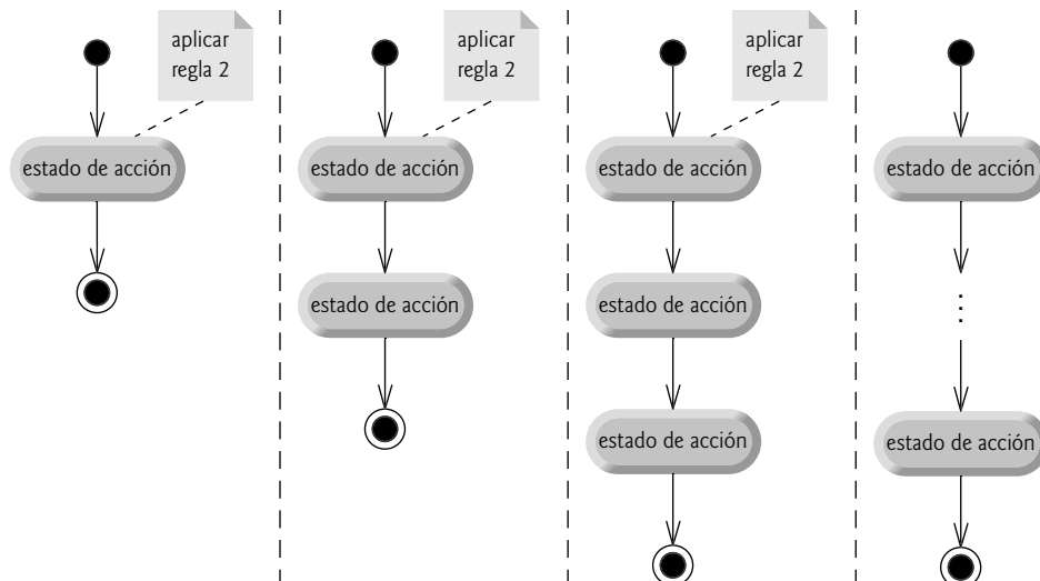
Fig. 5.24 | El resultado de aplicar la regla 2 de la figura 5.22 repetidamente al diagrama de actividad más sencillo.
