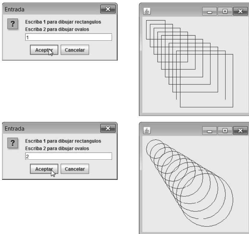
Fig. 5.28 | Cómo obtener datos de entrada del usuario y crear un objeto JFrame para mostrar Figuras (parte 2 de 2).
