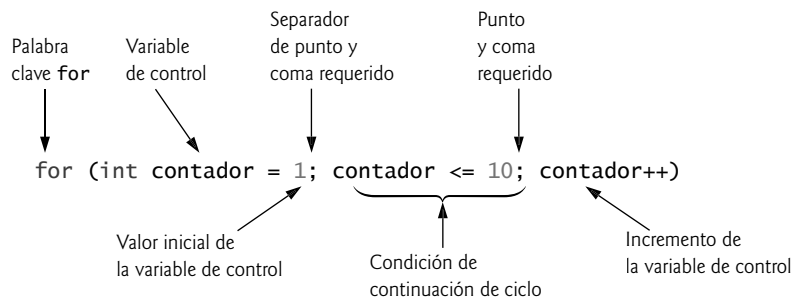
Fig. 5.3 | Componentes del encabezado de la instrucción for .
