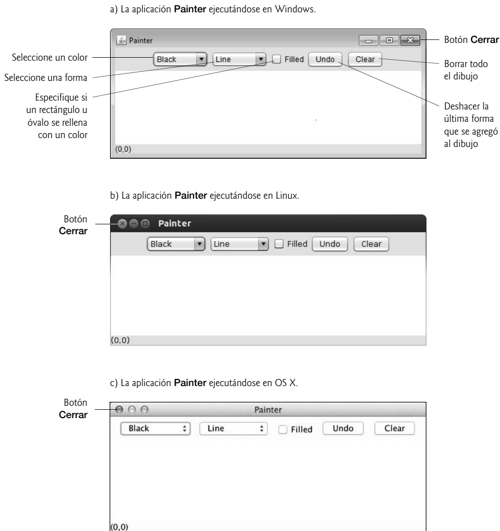
Fig. 1.11 | La aplicación Painter ejecutándose en Windows 7, Linux y OS X.
