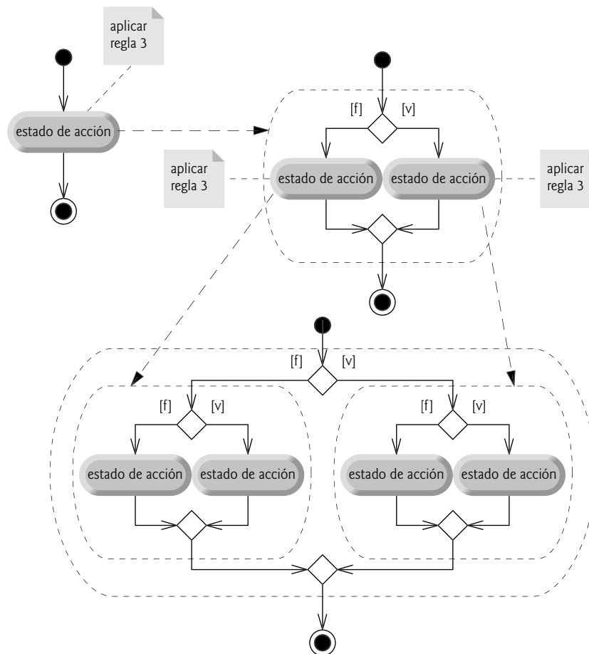
Fig. 5.25 | Aplicación en forma repetida de la regla 3 de la figura 5.22 al diagrama de actividad más sencillo.
