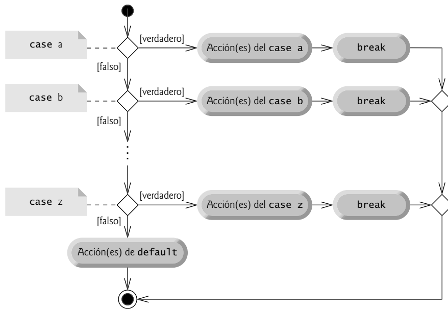
Fig. 5.10 | Diagrama de actividad de UML de la instrucción switch de selección múltiple con instrucciones break .
