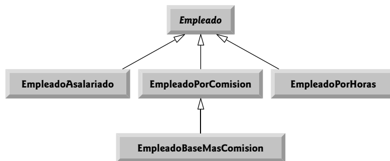
Fig. 10.2 | Diagrama de clases de UML para la jerarquía de Empleado .
