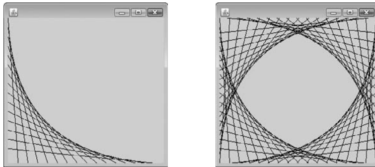
Fig. 4.21 | Arte lineal con ciclos y drawLine .
