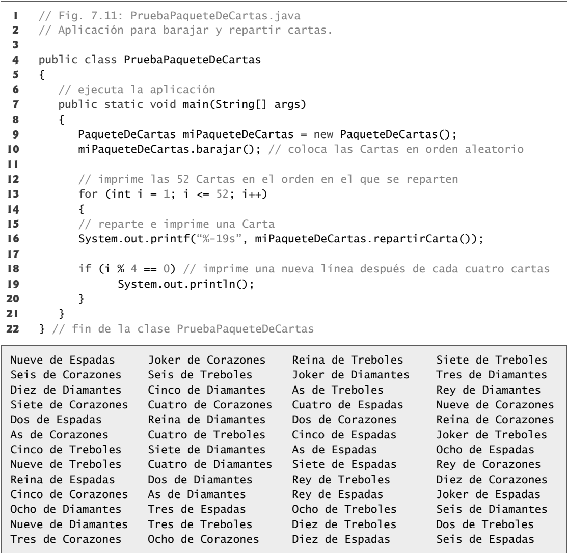
Fig. 7.11 | Aplicación para barajar y repartir cartas .
