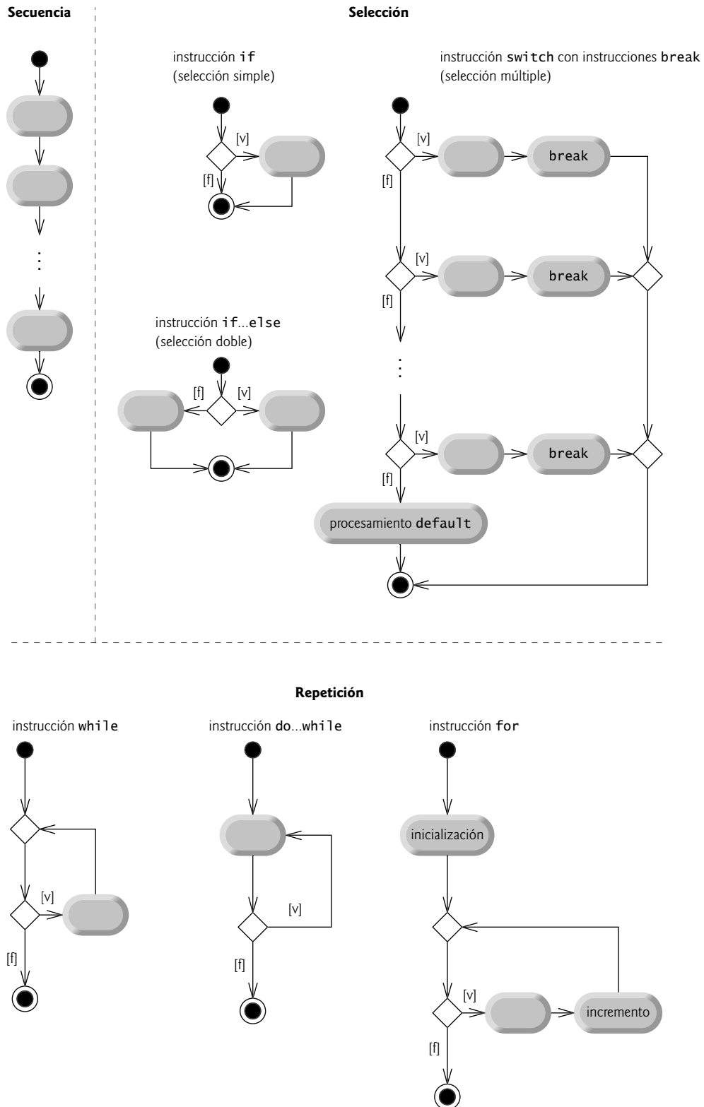
Fig. 5.21 | Instrucciones de secuencia, selección y repetición de una sola entrada/una sola salida de Java.
