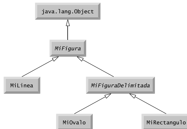
Fig. 10.18 | Jerarquía MiFigura con MiFiguraDelimitada .
